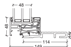
24mm alu/PA elementdybde 149mm og 174mm
