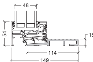
15mm komposit elementdybde 149mm og 174mm
